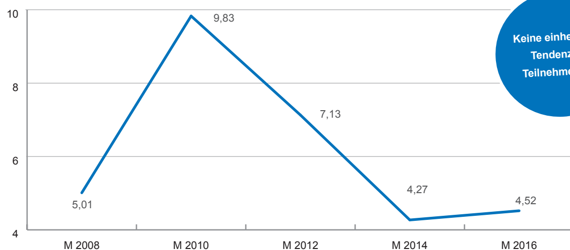
Entwicklung der Medianwerte (M) der kurzfristigen sanierungsbedürftigen Kanallängenrate (von 2008 bis 2016)
