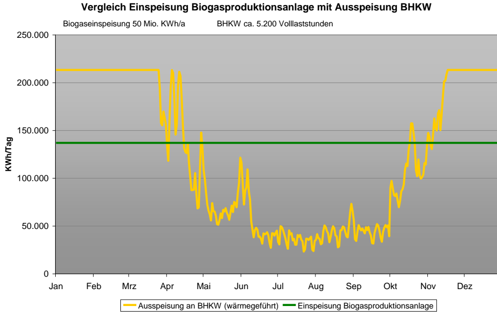
Abbildung 1 Beispiel für die Einspeisung aus einer Biogasproduktionsanlage und der Auspeisung an ein BHKW 1
