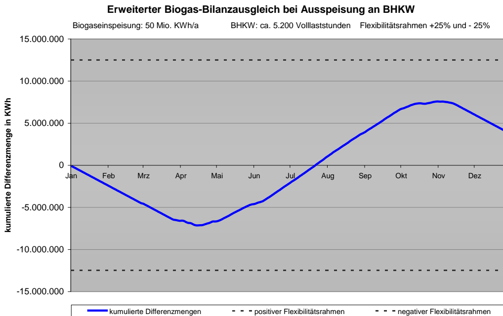
Abbildung 2 Erweiterter Biogas-Bilanzausgleich bei Auspeisung an BHKW
