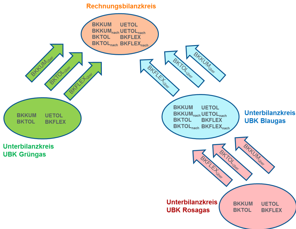
Abbildung 37: Kaskadische Bilanzkreiskonstruktion – Zeitreihen Untertägige Verpflichtung
