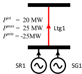
Abbildung 13: Exemplarische Flexibilitätsbeschränkung für mehrere Ressourcen
