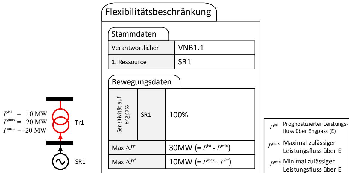
Abbildung 12: Exemplarische Flexibilitätsbeschränkung durch einen HS-/MS-Transformator
