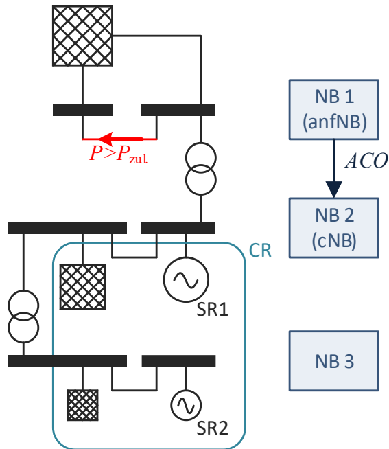
Abbildung 18: Skizze Netzkonstellation Szenario 1
