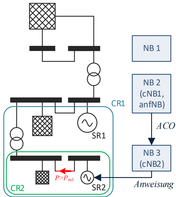
Abbildung 24: Skizze Netzkonstellation Szenario 4
