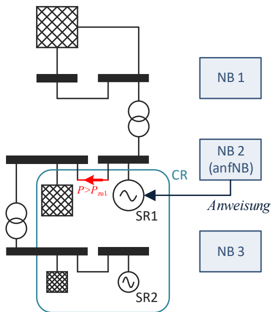
Abbildung 20: Skizze Netzkonstellation Szenario 2
