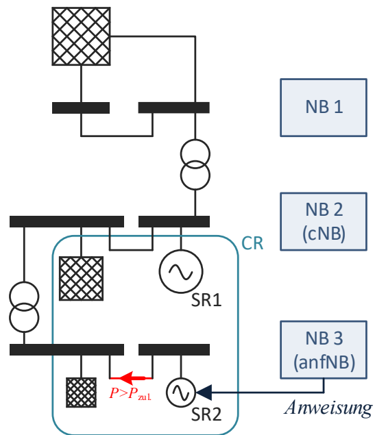
Abbildung 22: Skizze Netzkonstellation Szenario 3
